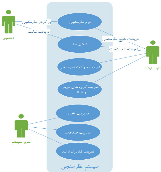
شکل (۴) نمودار Use Case سیستم نظرسنجی
